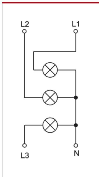
Принципиальная электрическая схема OptiDin FSL63
